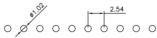
P.C.B LAYOUT
