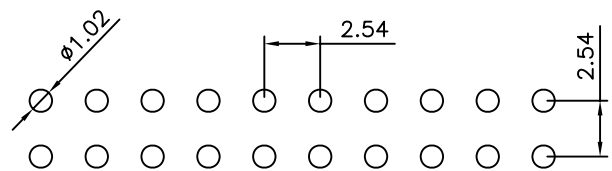
P.C.B LAYOUT
