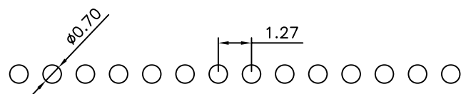
P.C.B LAYOUT
