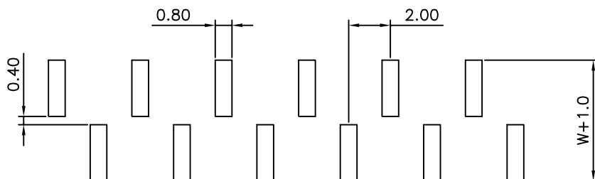
P.C.B LAYOUT
